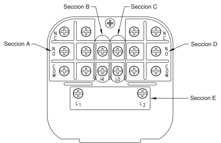
Figura 8 Placa de Terminales
