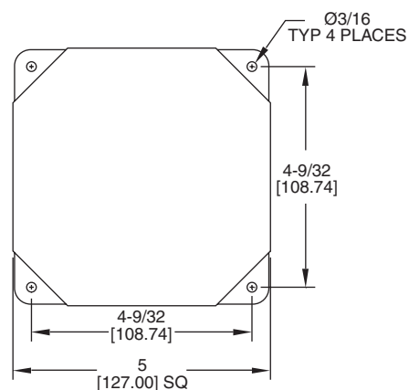
Figura 6 Esquema de los Agujeros
