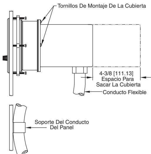
Figura 7 Detalles del Montaje
