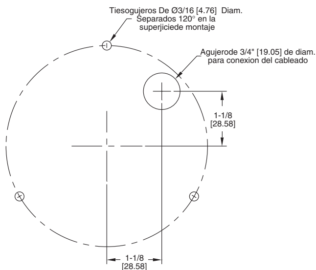
Figura 4 Esquema del Agujero (de frente)
